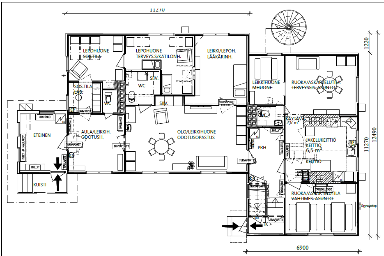
Rakennuksen pohjapiirros, 1. kerros. Yliviivattuna huoneiden alkuperäiset käyttötarkoitukset. Arkkitehtitoimisto Lindholm Oy 2020.
