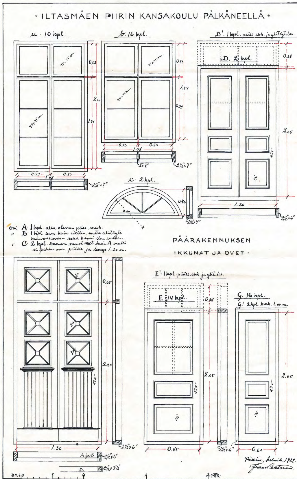
Päärakennuksen ikkuna- ja ovikaaviot. Lähde: Pälkäneen kunnan arkisto.
