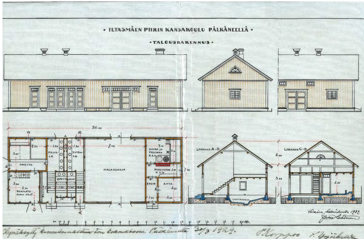
Iltaasmaen koulun talousrakennuksen piirrokset vuodelta 1929. Lähde: Pälkäneen kunnan arkisto.
