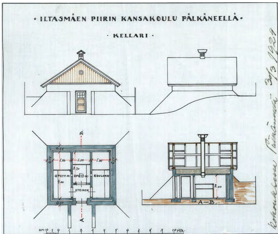
Iltaasmaen koulun kellarin piirustukset vuodelta 1929. Lähde: Pälkäneen kunnan arkisto.
