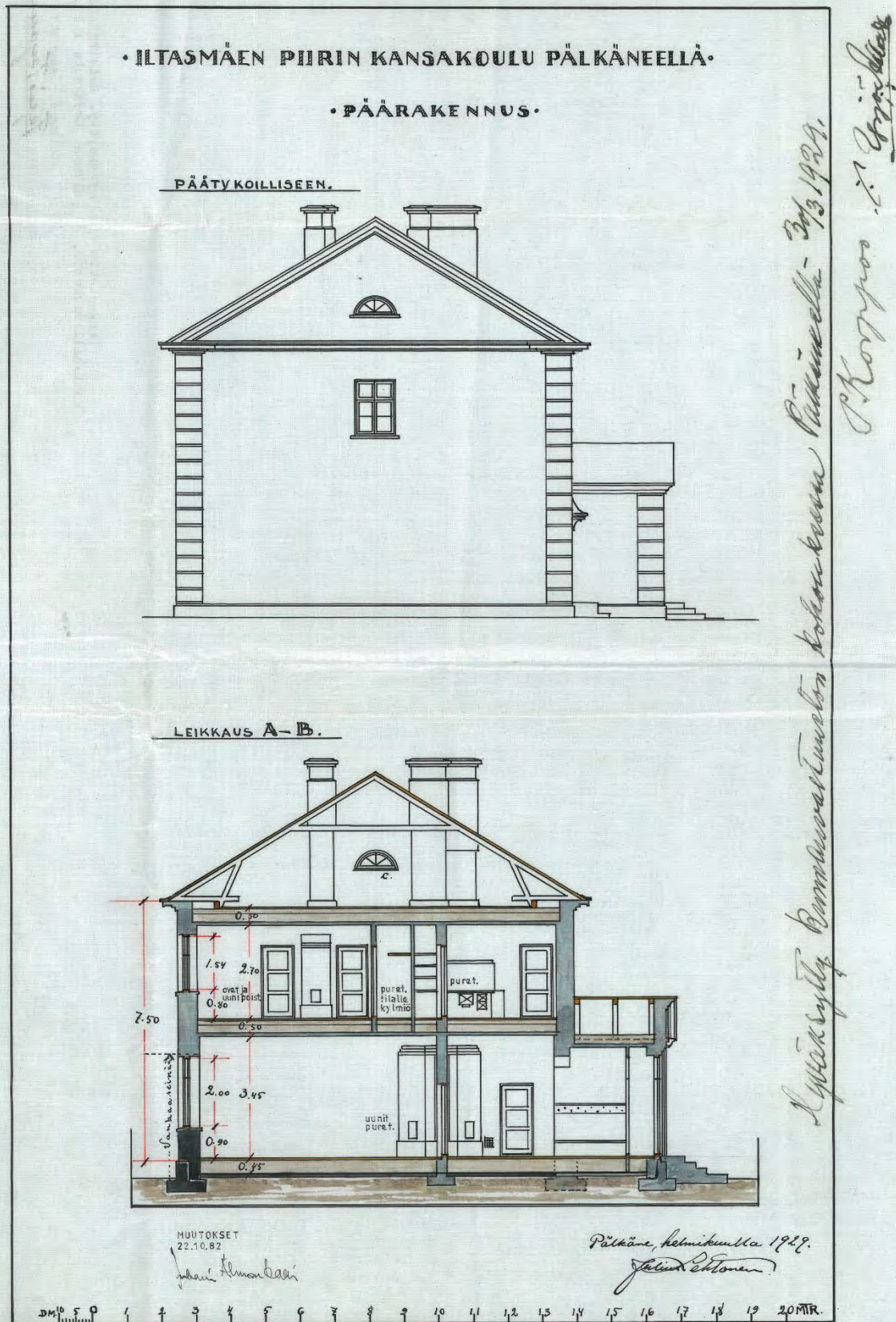
Ilta-Mäen koulun julkisivu koilliseen ja leikkauspiirustus vuodelta 1929.
