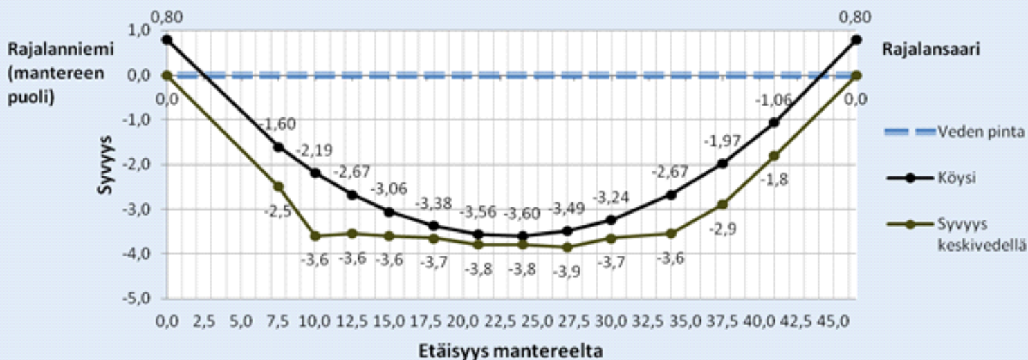
Vähäsalmen syvyyskäyrä ja lossiköyden mallintaminen
